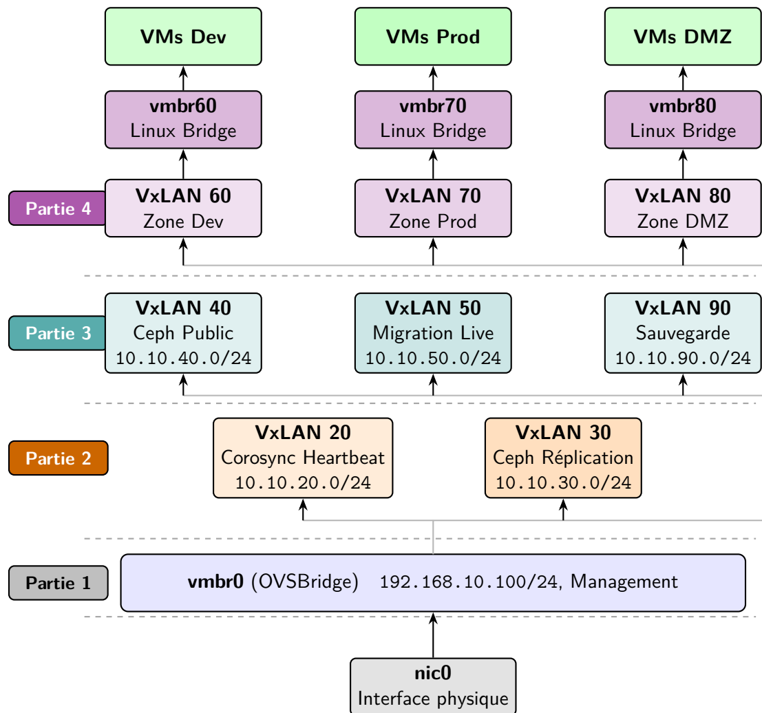
FIGURE IV.44 – Vue d'ensemble de la configuration réseau de PVE-01 : quatre parties logiques
